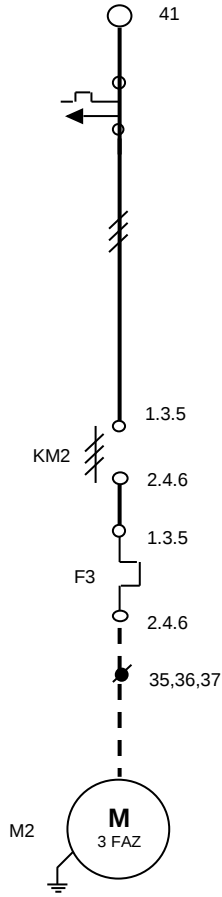
POMPA MOTORU
