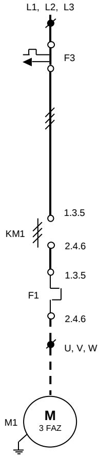
FAN MOTORU
